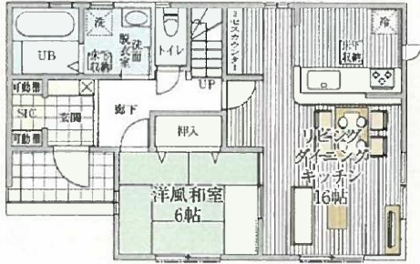
完成予想図
